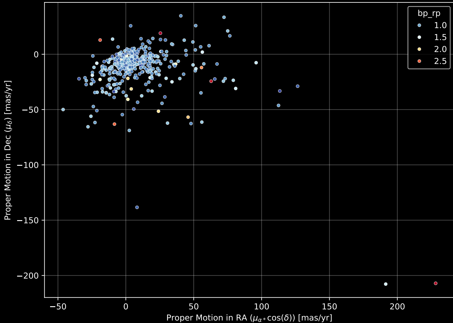
GALAH DR4 Field: [6696] Proper Motion Diagram (n= 399)
