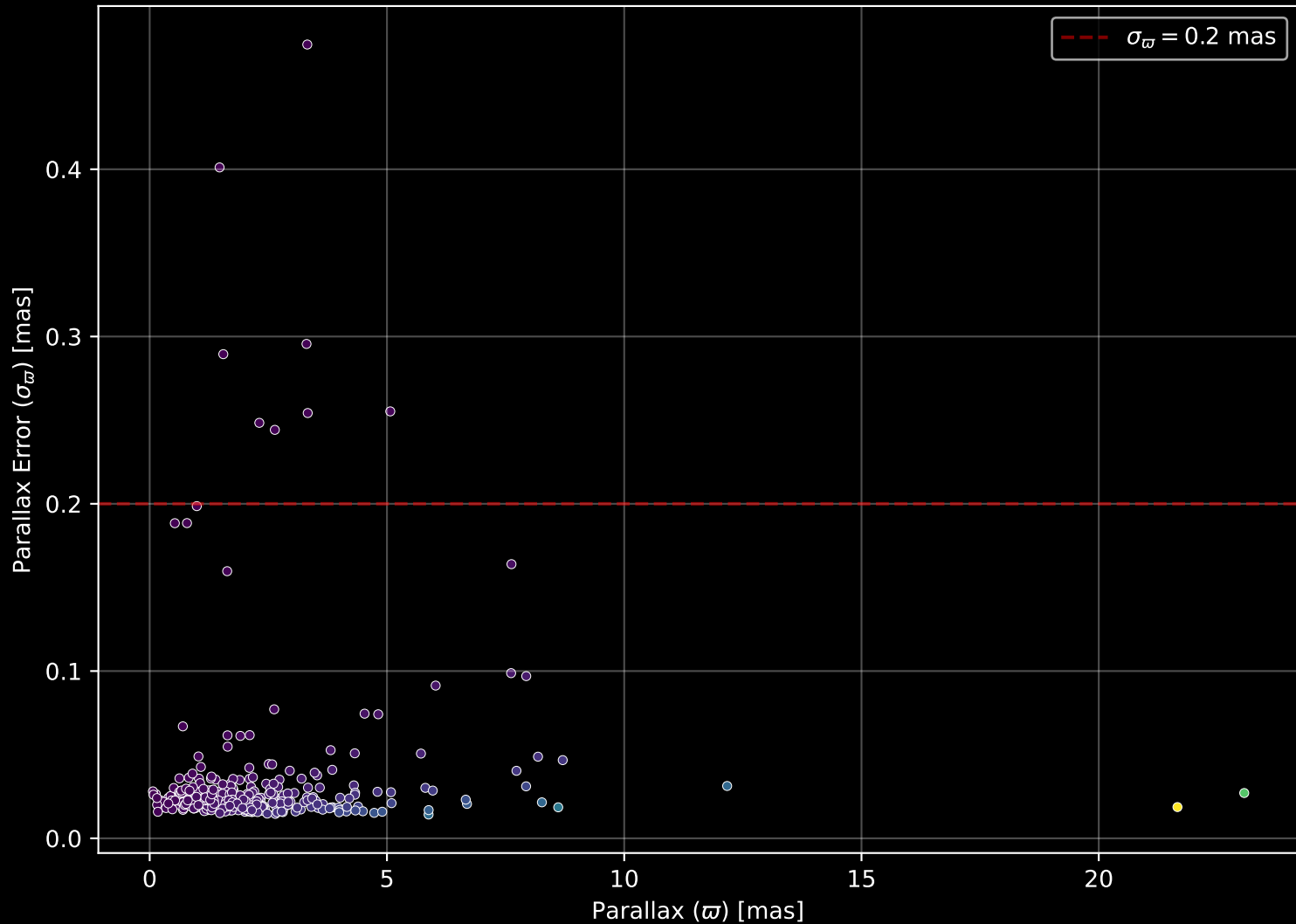
GALAH DR4 Field: [6696] Parallax Quality (n= 399)
