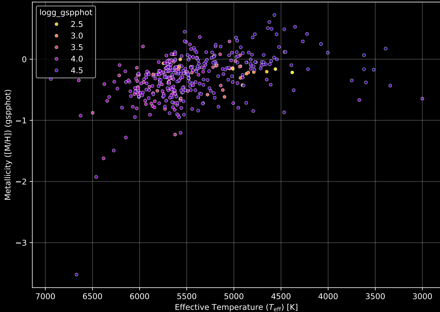
GALAH DR4 Field: [6696] Stellar Population Parameters (n= 399)
