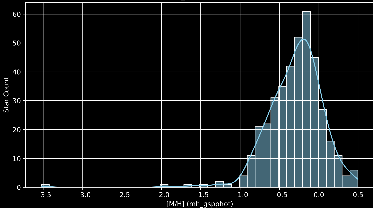
GALAH DR4 Field: [6696] [M/H] (mh_gspphot) (n= 395)
